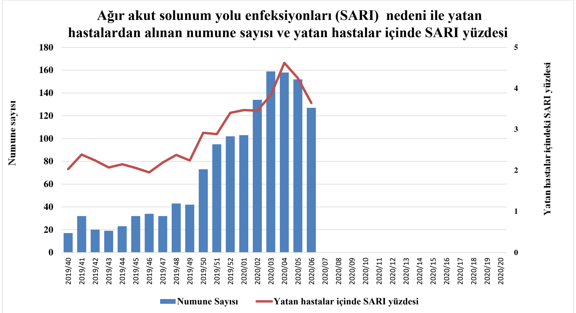
Grafik-3: Sentinel Ağır Akut Solunum Yolu Enfeksiyonları (SARI) Sürveyansı kapsamında haftalık çalışılan Ağır Akut Solunum Yolu Enfeksiyonları (SARI)numune sayısı ve yatan hastalar içinde SARI yüzdesi.
